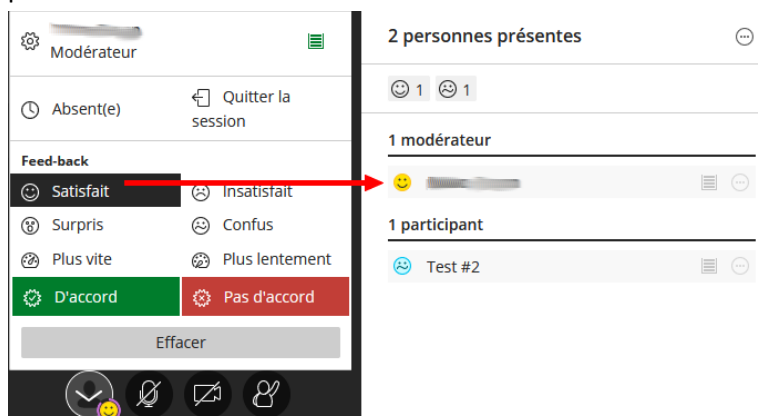
Sélection d'un émoticône de de Feed-back et son rendu dans la fenêtre des Personnes présentes
